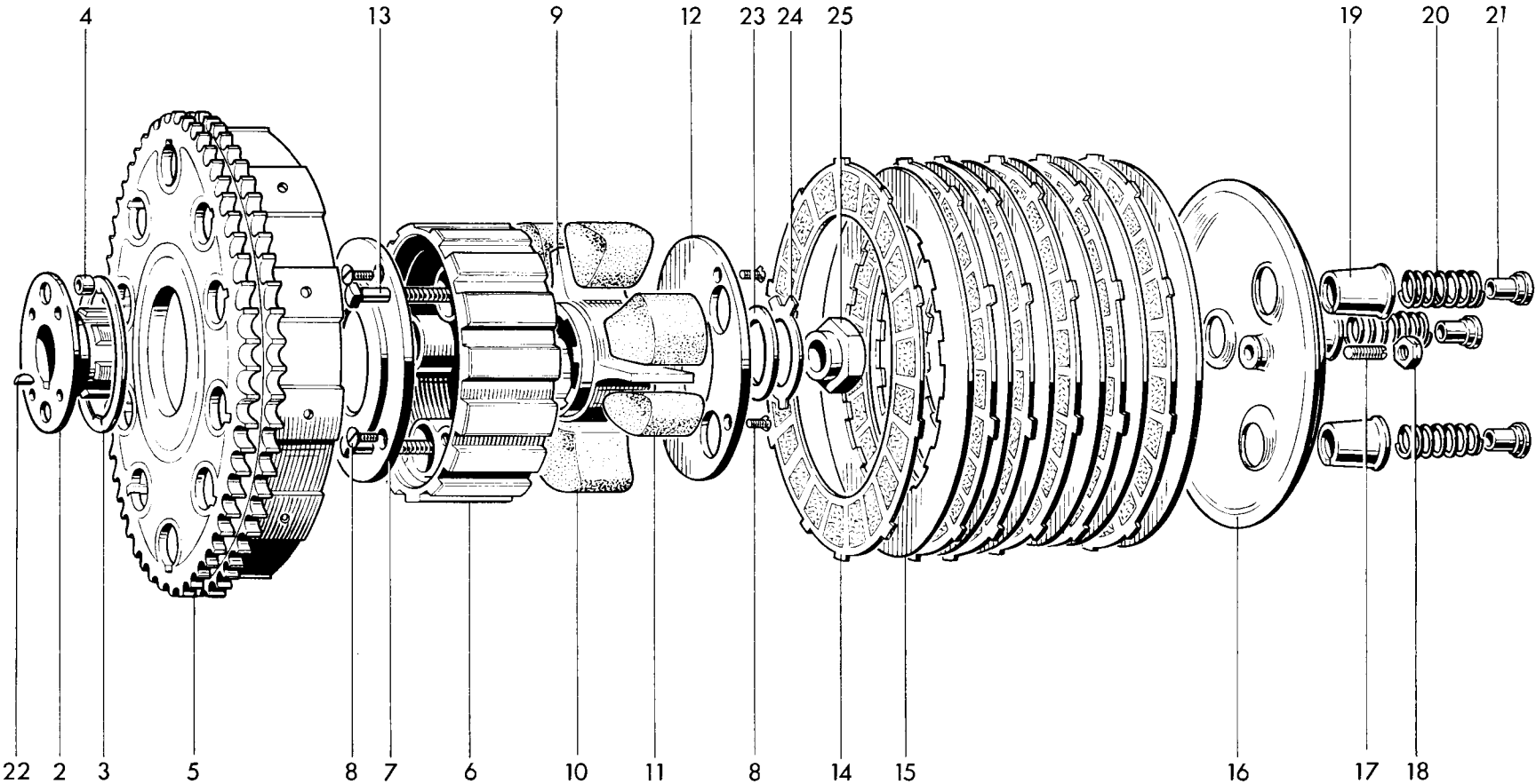
Fig. 10. CLUTCH
