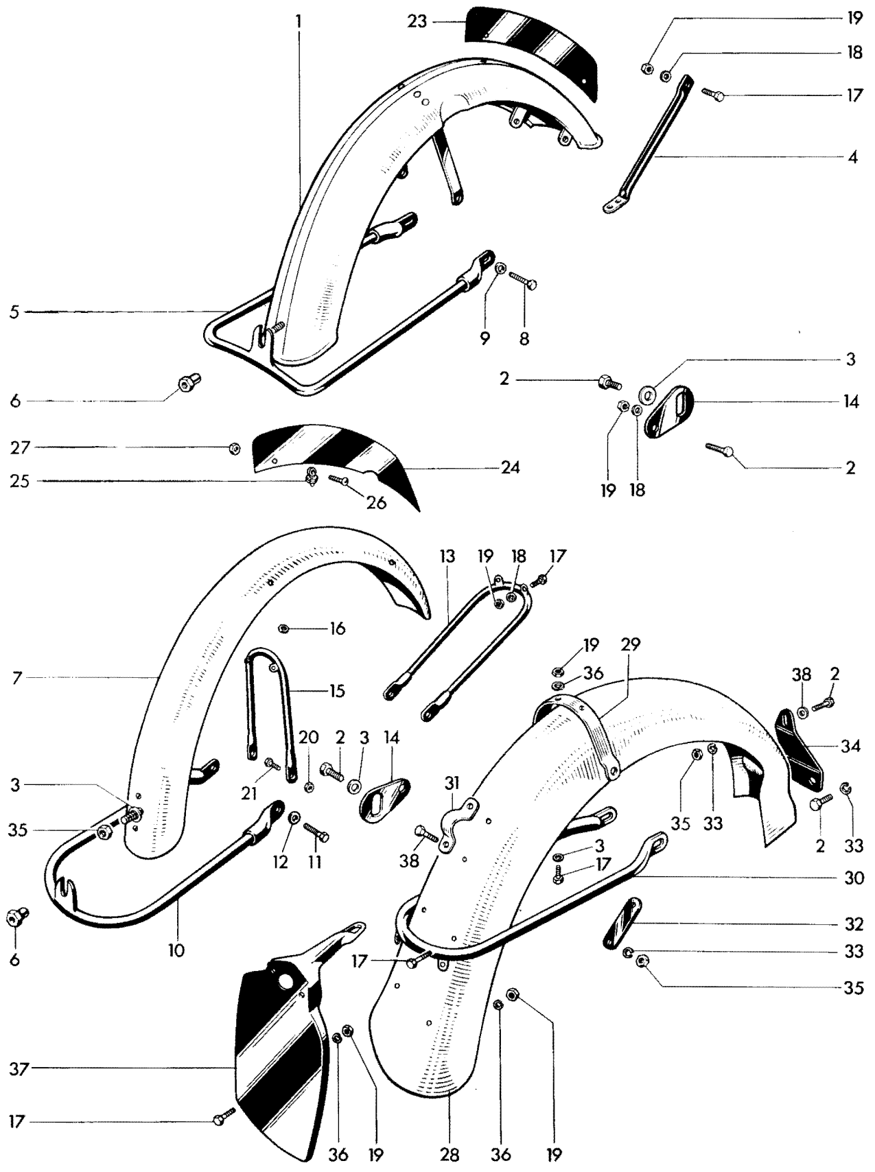
Fig. 29. MUDGUARDS (STANDARD)
