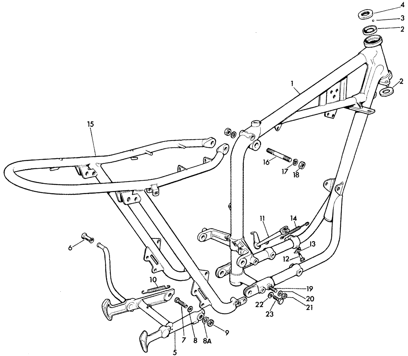
Fig. 12. FRAME
